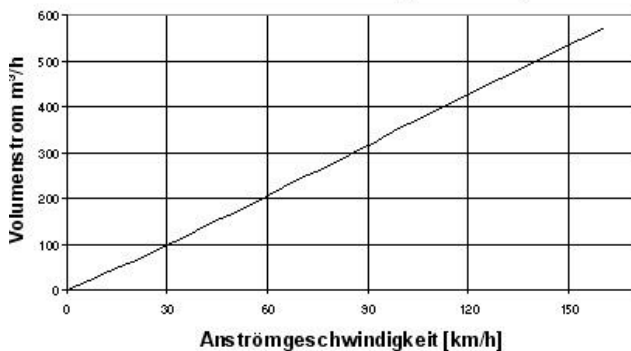
Volumenstrom bei Anströmgeschwindigkeit
