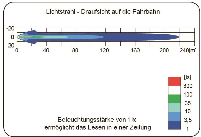
(Spotausführung LED-AS5F)
