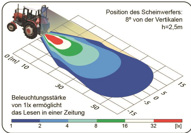
(Standardausführung LED-A5F)
